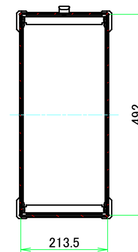
C-C ( 1 : 9.5 )
