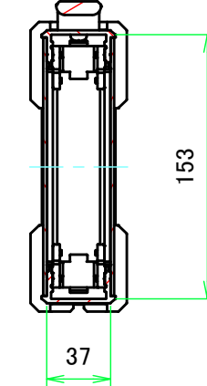
C-C ( 1:4 )
