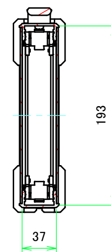
C-C ( 1:4 )
