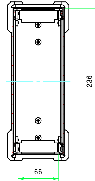
A-A ( 1:3.5 )
