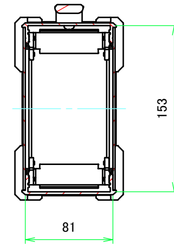
C-C ( 1:3.5 )
