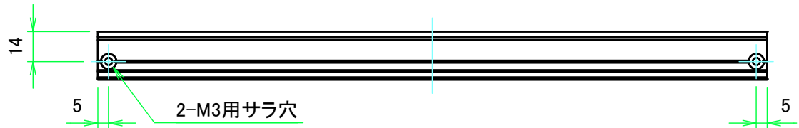
2-M3用サラ穴 2-M3 Countersunk ※ 反対面も同様 / Same on the other side.
