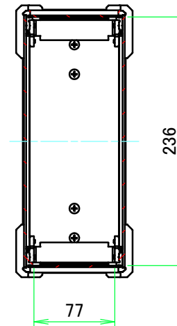
A-A (1:5)
