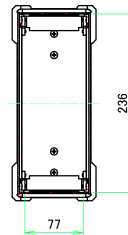
A-A (1:5)
