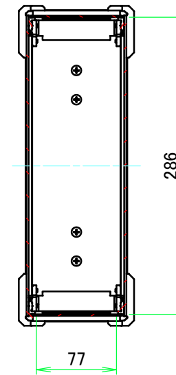
A-A (1:5)
