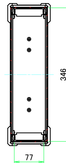
A-A (1:6)
