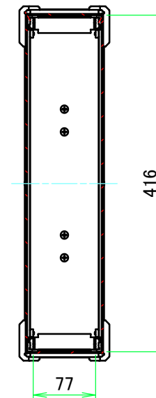
A-A (1:6.5)
