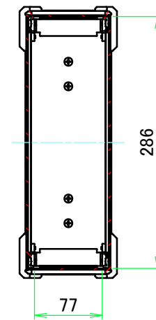
A-A (1:6)
