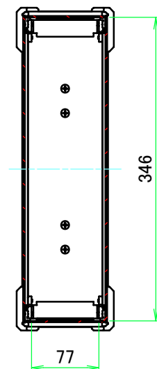
A-A ( 1 : 6 )
