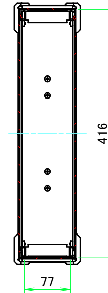
A-A ( 1 : 6.5 )
