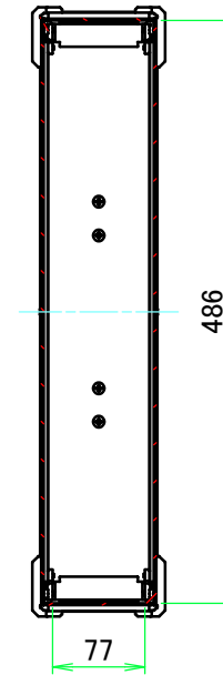
A-A (1:7)
