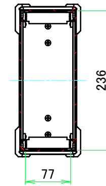
A-A (1:6.5)
