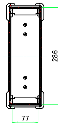
A-A (1:6.5)
