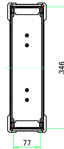
A-A (1:6.5)
