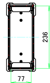
A-A ( 1 : 7.5 )
