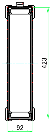
C-C ( 1 : 7.5 )
