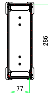
A-A (1:7.5)
