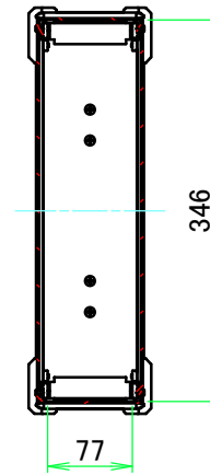
A-A (1:7.5)
