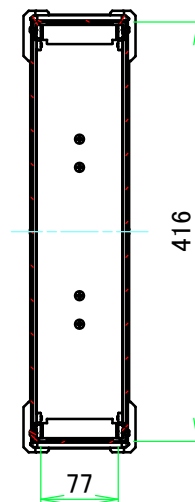
A-A (1:7.5)
