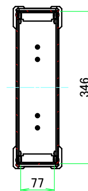
A-A (1:8.5)
