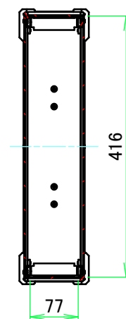
A-A (1:8.5)
