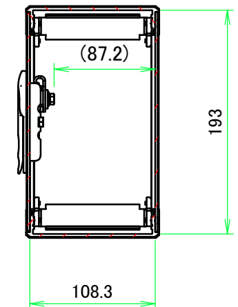
B-B ( 1 : 4.5 )
