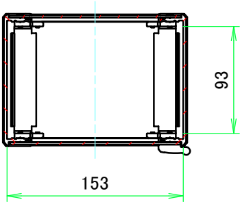
A-A ( 1 : 4.5 )
