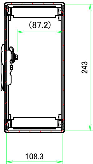
B-B ( 1 : 4.5 )
