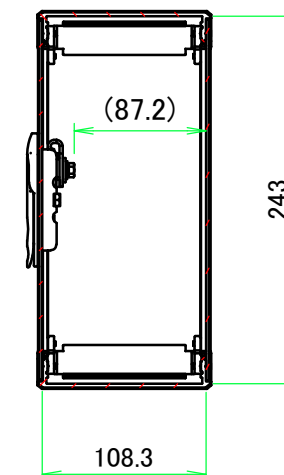
B-B ( 1 : 5 )
