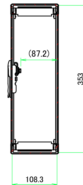
B-B ( 1 : 5.5 )
