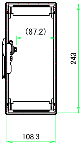
B-B ( 1 : 5 )
