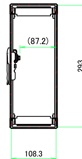
B-B ( 1 : 5.5 )
