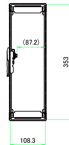
B-B ( 1 : 6 )
