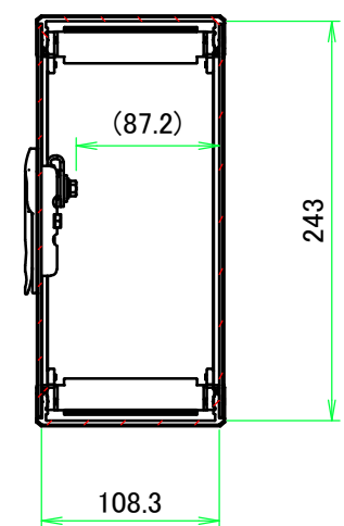
B-B ( 1 : 5 )
