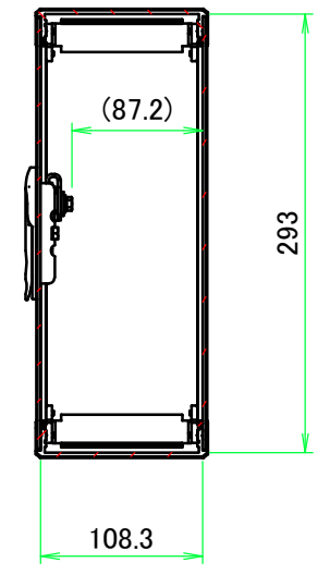
B-B ( 1 : 5.5 )
