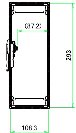
B-B ( 1 : 5.5 )
