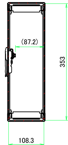
B-B ( 1 : 6 )
