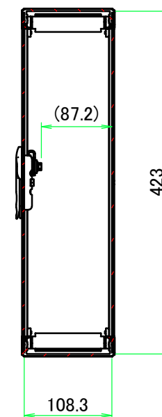
B-B ( 1 : 6.5 )
