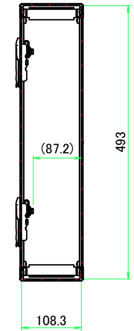
B-B ( 1 : 7 )
