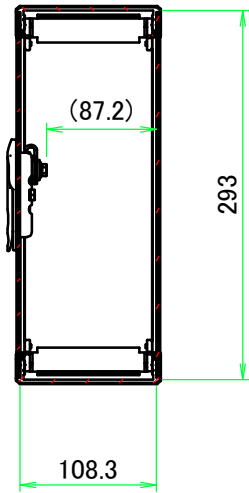
B-B ( 1 : 6 )
