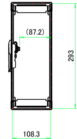
B-B ( 1 : 6 )
