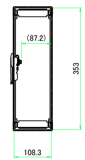
B-B ( 1 : 6.5 )
