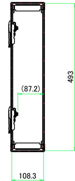
B-B ( 1 : 7.5 )
