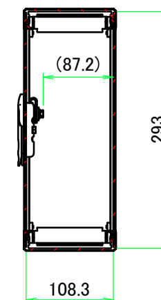
B-B ( 1 : 6.5 )
