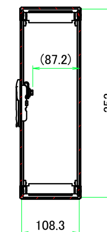
B-B ( 1 : 7 )
