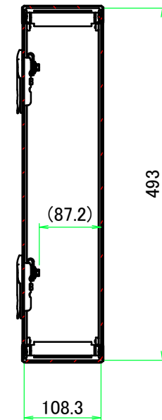
B-B ( 1 : 7.5 )
