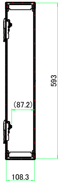
B-B ( 1 : 8.5 )
