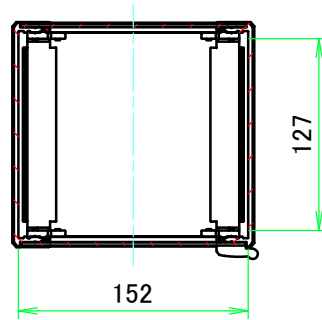
A-A ( 1 : 5 )
