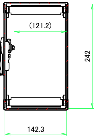
B-B ( 1 : 5 )
