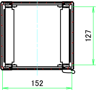
A-A ( 1 : 5 )
