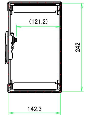
B-B ( 1 : 5 )
