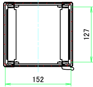
A-A ( 1 : 5 )
