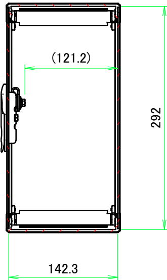
B-B ( 1 : 5 )
