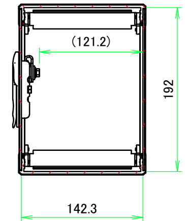
B-B ( 1 : 4.5 )
