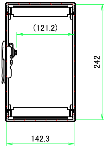
B-B ( 1 : 5 )
